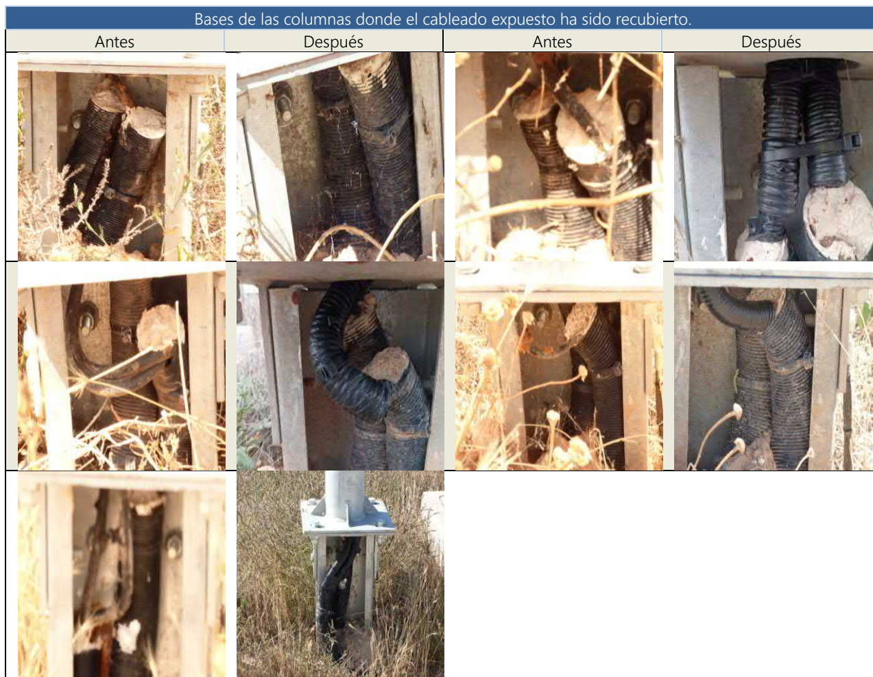
Imágenes 6, 7, 8, 9, 10, 11, 12, 13, 14 y 15: bases de las columnas antes y después de la protección del cableado
